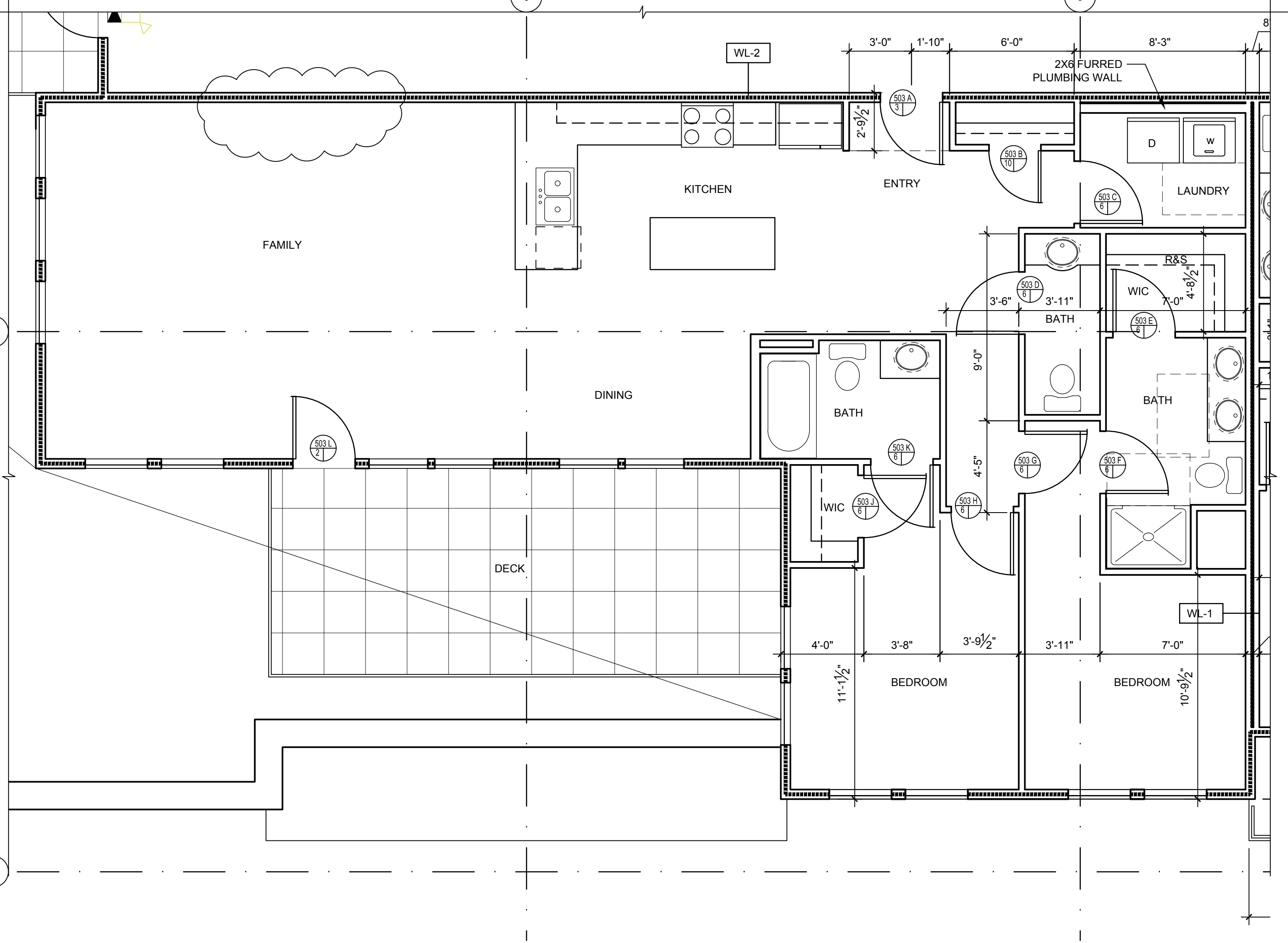
1 UNIT 503 SCALE: 1/4"=1'-0"
