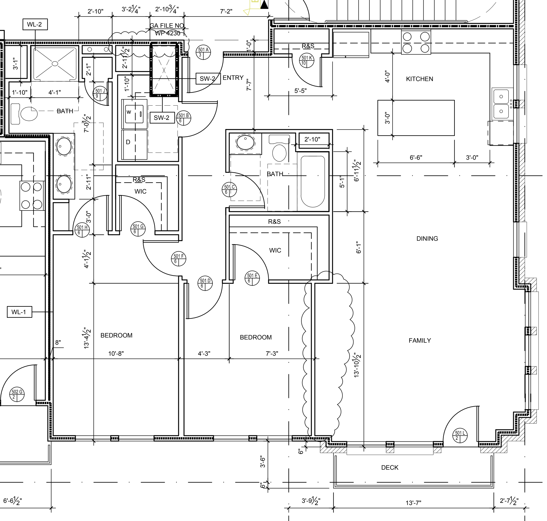
2 UNIT 501 SCALE: 1/4"=1'-0"
