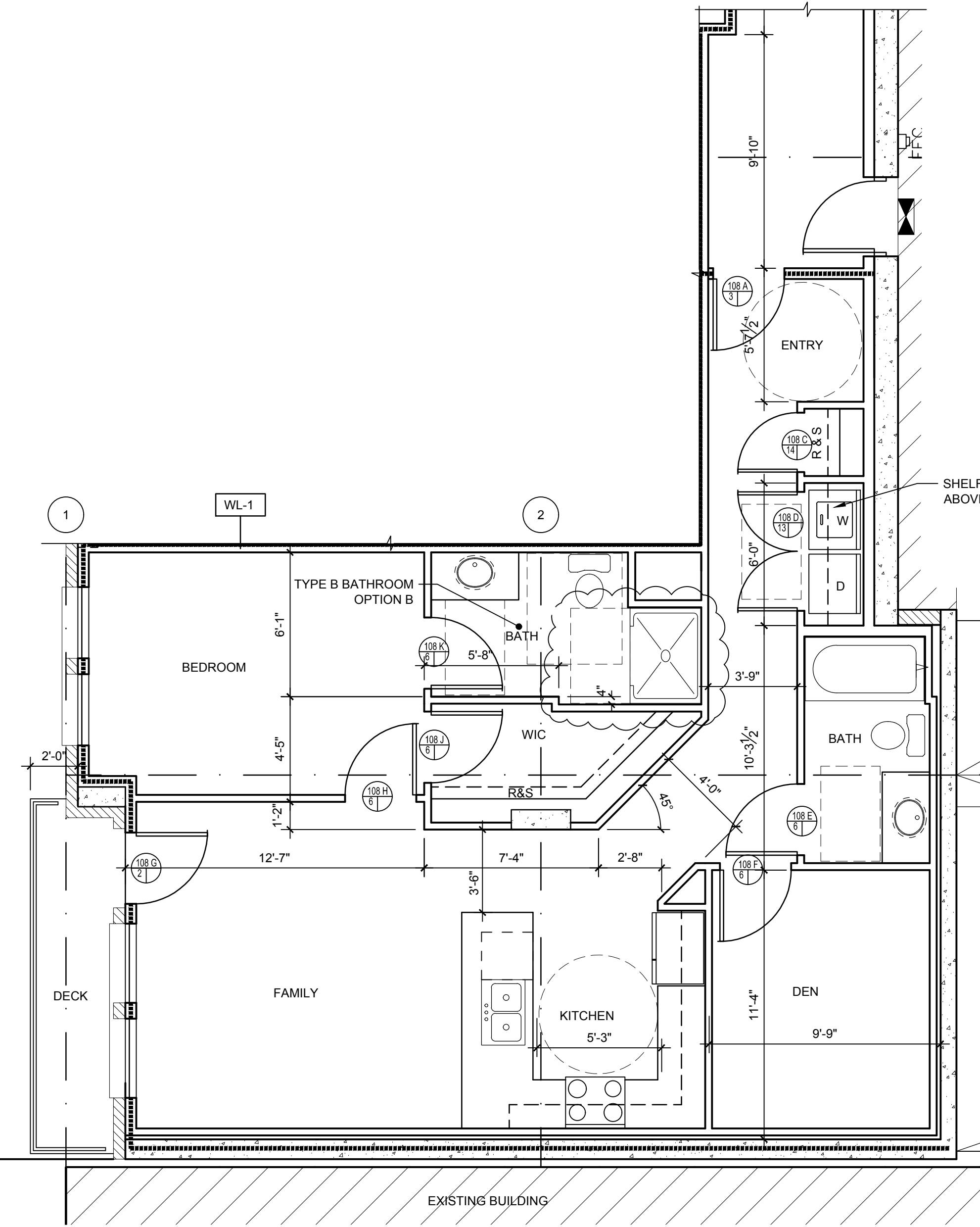
1 UNIT 108 SCALE: 1/4"=1'-0"
